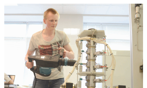
В насыпной модели можно задавать необходимые свойства пласта, а затем изучать происходящие в нем процессы.
