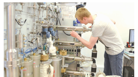
Образец направляется в «шкаф» установки для исследования кернa, где создается необходимая температура.
